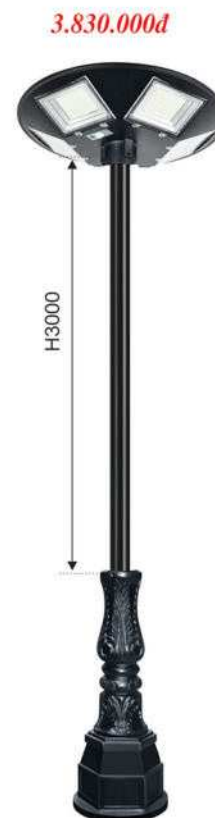
SOLAR - TRỤ 157 Ø Đèn: 550 x H125 - ABS Ø Đế: 300 x H3700 BNL: 6V - 25W - Pin : 30 AH Bóng phát sáng 300W Cảm biến ánh sáng - IP65 Thấp sáng: 8 -> 10 giờ 10.330.000đ ○●
