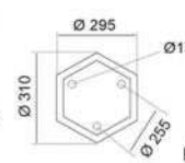
TRỤ 292 L800 x H4000 E27 x 3 13.600.000đ
