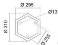
TRỤ 288 L800 x H4000 E27 x 3 14.000.000đ
