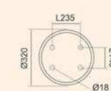
CHÂN ĐẾ 15 H1180 - Nhôm 8.730.000d
