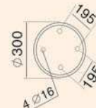
CHÂN ĐẾ 05 H1000 - Nhôm 3.780.000d
