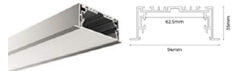
Thanh Profile 3594 PFVL-3594S/ PFVL-3594B/ PFVL-3594W
