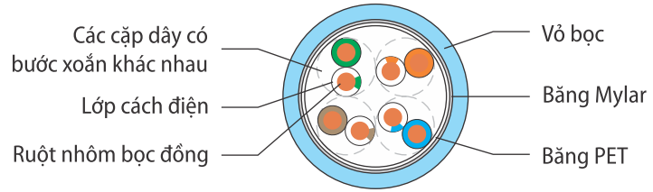
FTP/CAT5E/VL/CCA/XN
