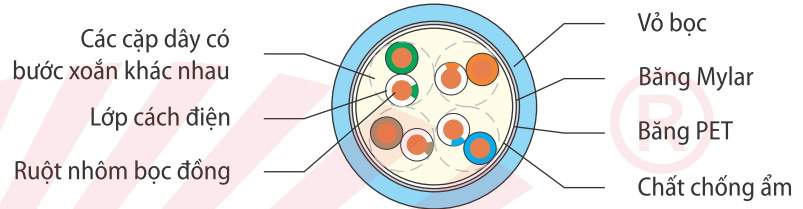
FTP/CAT5E/VL/CCA/CA/XN
