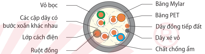
FTP/CAT5E/VL/CA
